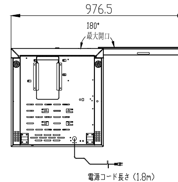
△1 底面図および扉開寸法追加
