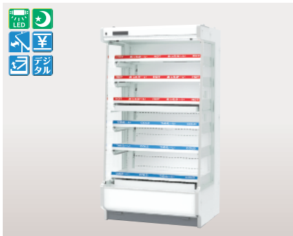
J-8 FDZ-HC32MNA 受注生産 外形寸法 幅915×奥行870×高さ1,900 陳列段数 7段全段加温機構付き 電源 単相100V・200V 50/60Hz 消費電力 (コールド時)47/47W (オールホット時)2,643W 質量 約217kg CO 2 569 ℓ
